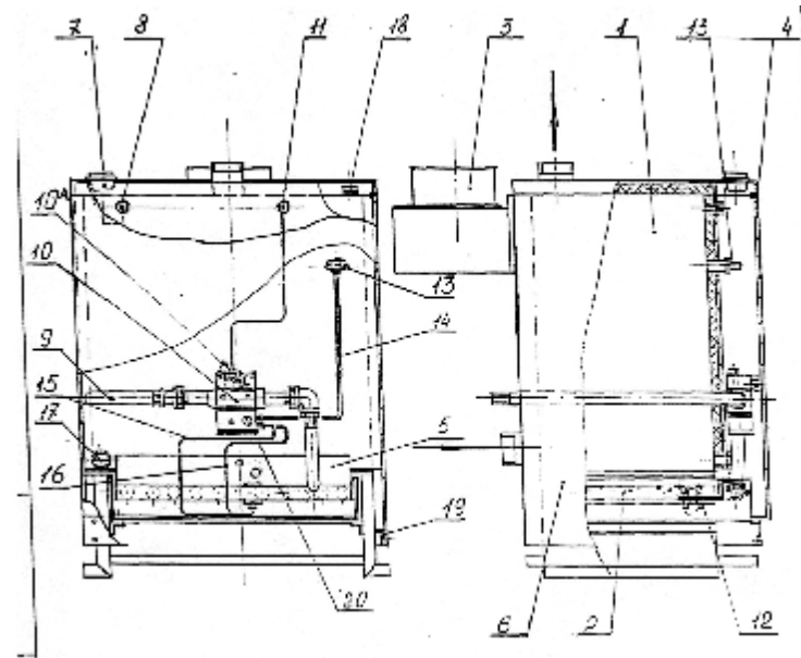
Рис.2. Конструкция котла
