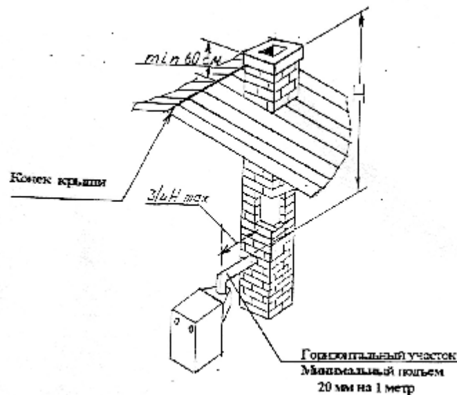
Рис. 7. Типовой кирпичный дымоход
