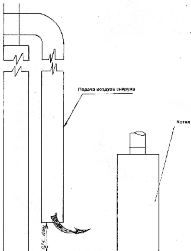
Рис.6 Поддача воздуха в герметично закрытое помещение
